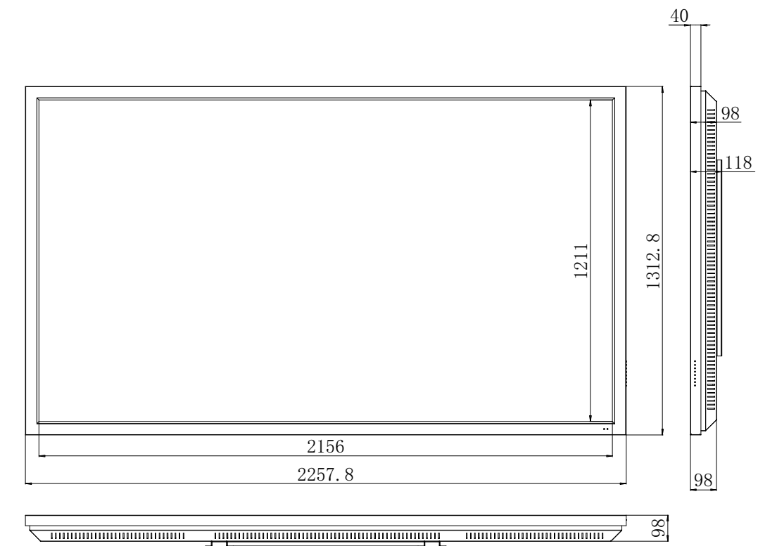
98寸监视器 总装图
